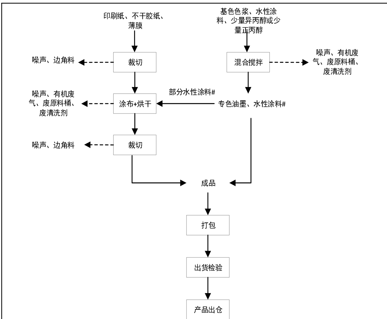
图2-1 生产工艺流程图
