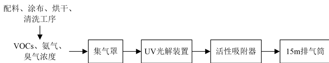
图3-2 项目废气处理流程图
